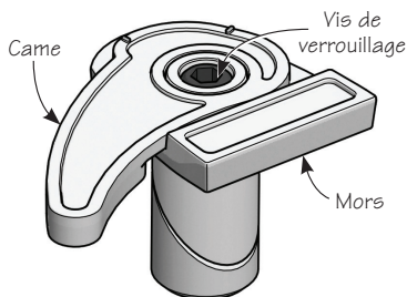
Figure : Composants du mentonnet à came
